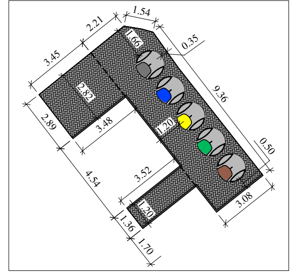
Aikštelės detalizacija
