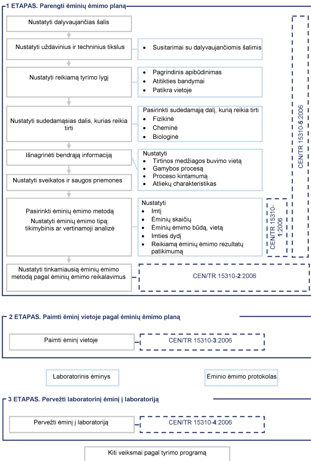
22 pav. Pagrindiniai ėminių ėmimo metodikos elementai pagal EN 14899:2005
