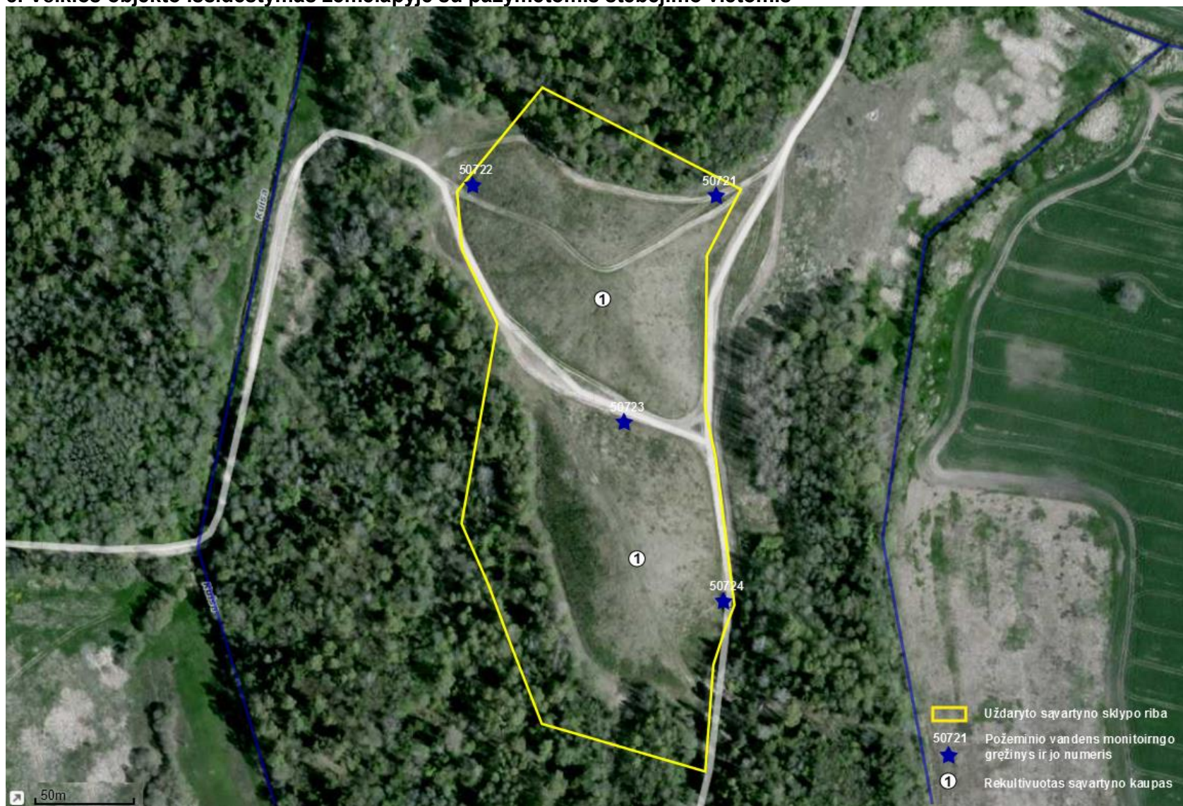
2 pav. Uždaryto Kuršėnų sąvartyno teritorijos planas su nurodytomis aplinkos monitoringo vietomis [7].
