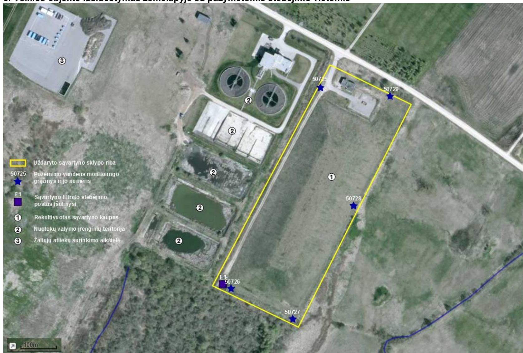
2 pav. Uždaryto Radviliškio KBA sąvartyno teritorijos planas su nurodytomis aplinkos monitoringo vietomis [8].
